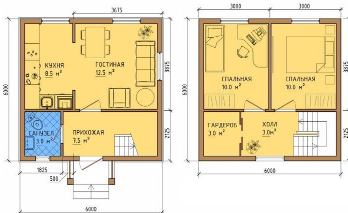
ПЛАНЫ ЭТАЖЕЙ
