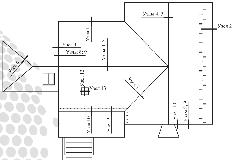
Рисунок А.11.1 - План крыши коттеджа и нумерация узлов
