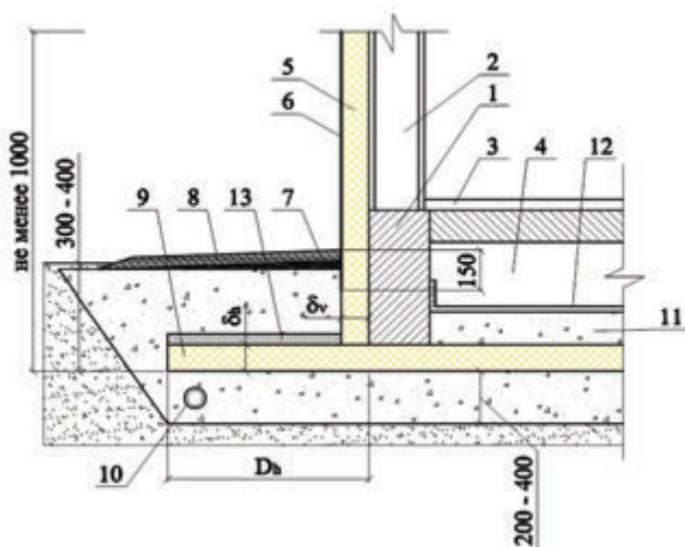
Рисунок 8.5.4. Схема укладки и параметры теплоизоляции в фундаментах зданий с неветилируемым подпольем и переменным режимом эксплуатации (отапливаемое – неотапливаемое)
