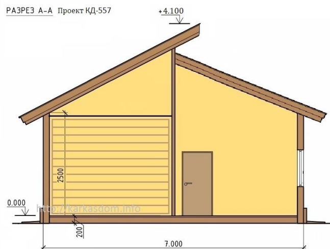
РАЗРЕЗ А-А Проект КД-557
