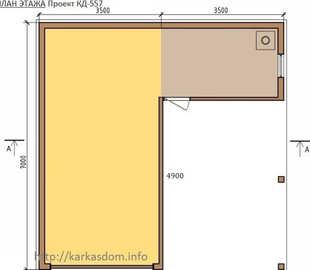
ПЛАН ЭТАЖА Проект КД-557
