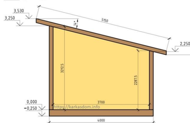
РАЗРЕЗ Проект КД-557
