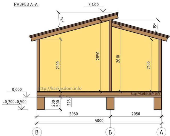
РАЗРЕЗ А-А.
