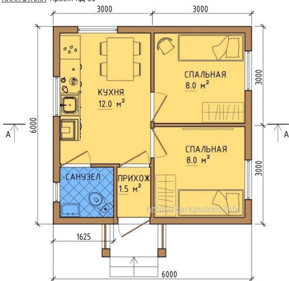
ПЛАН ЭТАЖА Проект КД-31
