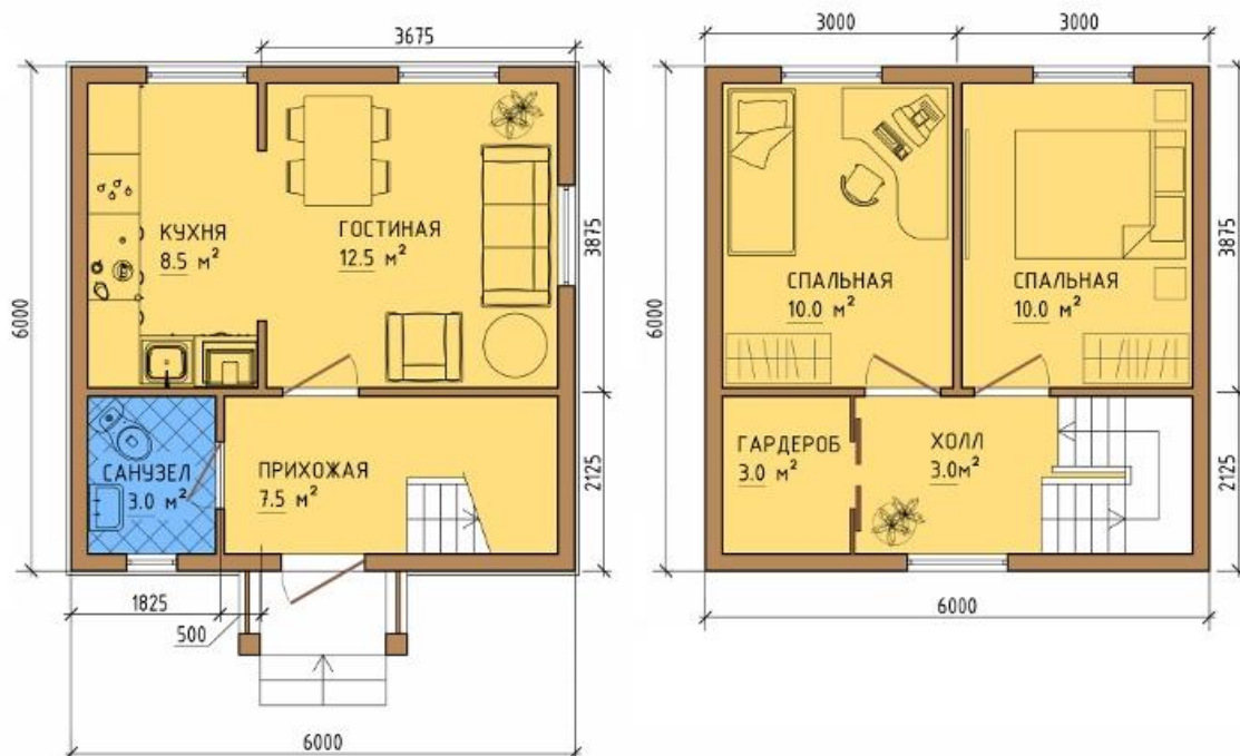
ПЛАНЫ ЭТАЖЕЙ
